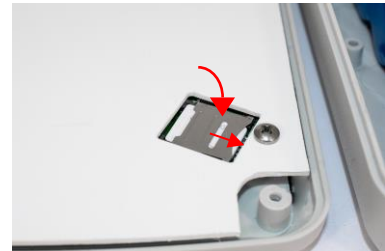
Halter verschließen
